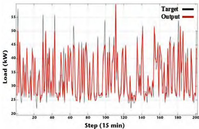
Abb. 1: Ist-Soll Diagramm für Testdaten bei wöchentlicher Lastvorhersage, Abbildungen: Ali Hashemifarzad, CUTEK
