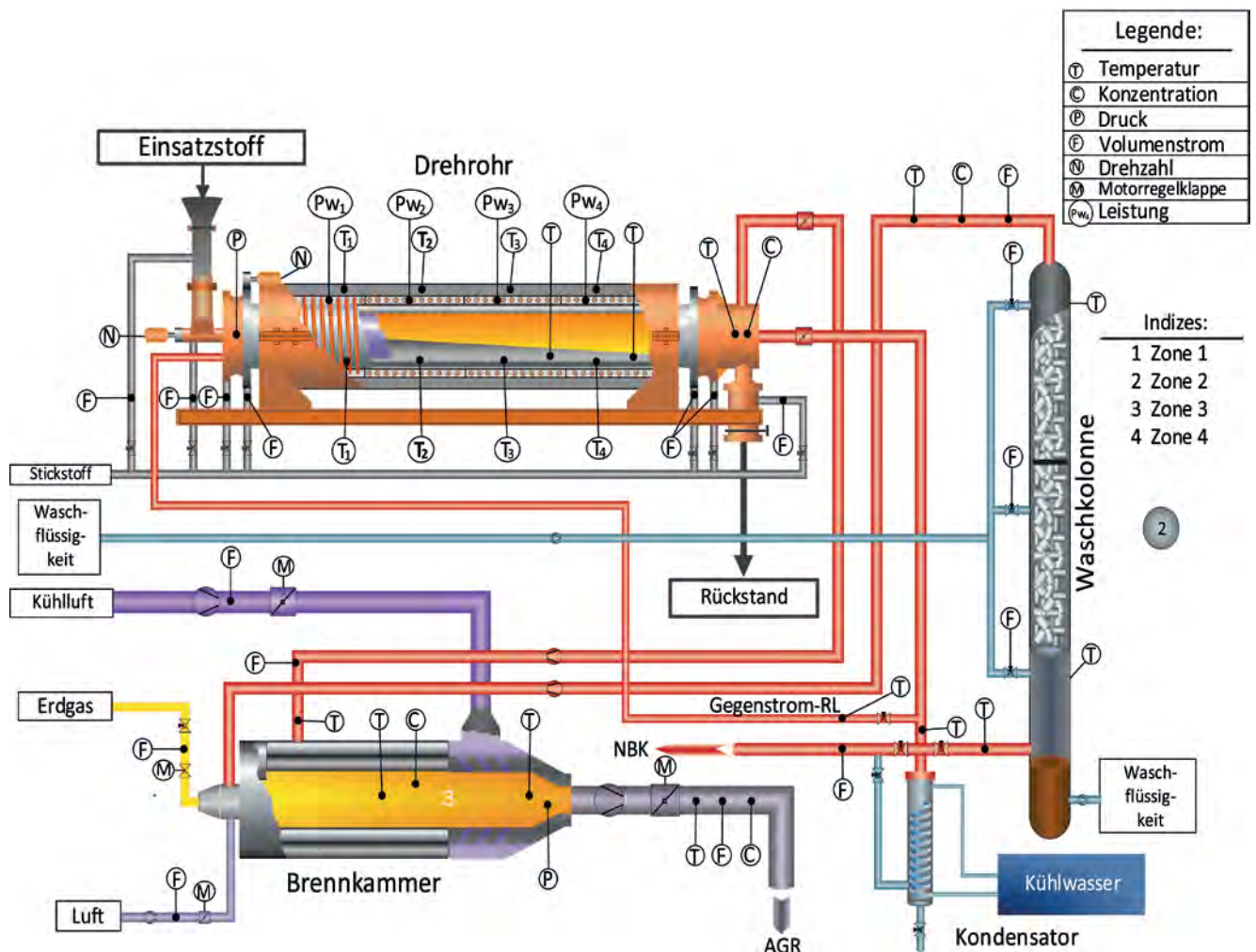
Abb. 1: Schematische Darstellung des Pyrolysedrehrohrs des CUTEC, Quelle: CUTEC, Abt. TP AGR: Abgasreinigung, NBK: Nachbrennkammer, RL: Rückleitung
