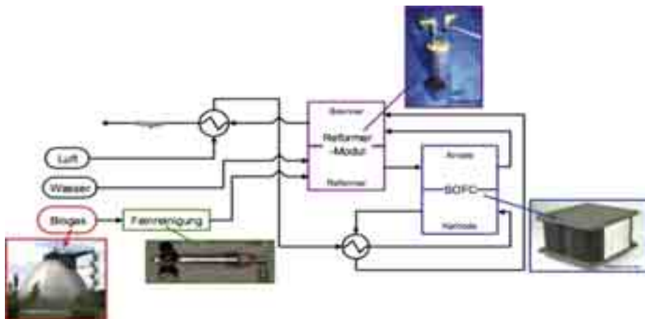
Schema des Systemaufbaus mit den Hauptgruppen
