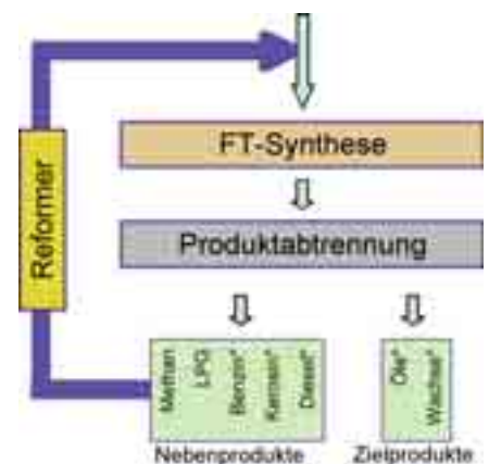
Abb. 3: FT - Wachssynthese mit Nebenprodukt-Rückführung zum Reformier (*Veredlung vor Vermarktung erforderlich)
