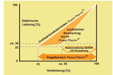
Leistungsbereich des Drehzahl modulierenden PowerTherm-BHKW im Vergleich zu herkömmlichen BHKW mit Drosselung
